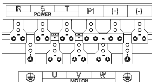
Схема силовых клемм для AP2-K25 ~ AP2-K35
