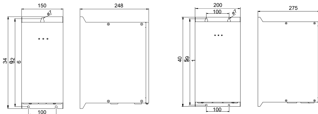
Габаритный чертеж BM10 - BM20
