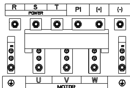
Схема силовых клемм для AP2-K16 ~ AP2-K22
