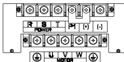
Схема силовых клемм для AP2-900 ~ AP2-K13
