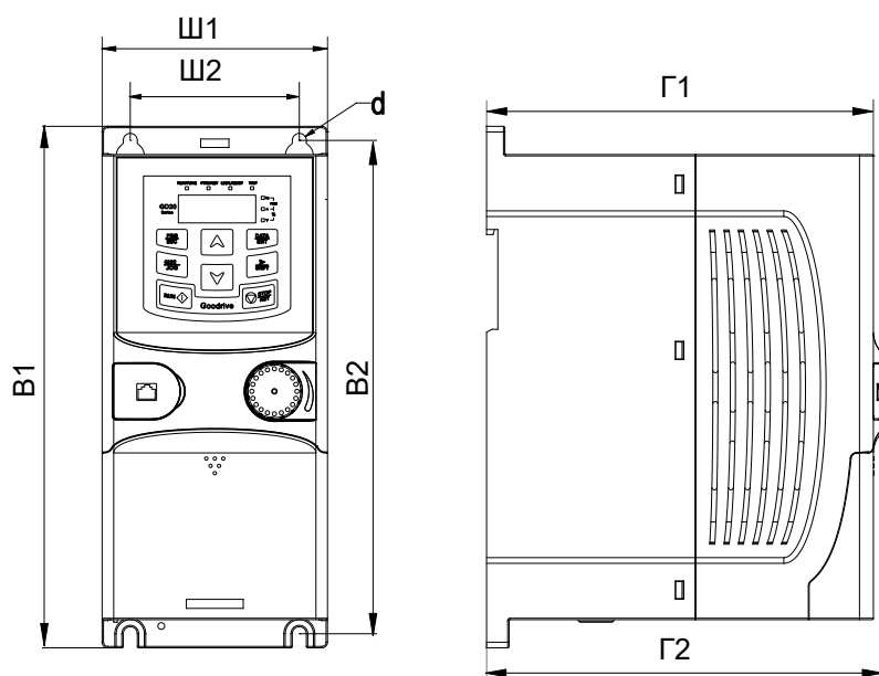
Размеры для настенного монтажа, AL-015B ~ AL-037B
