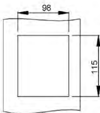
Установочные размеры
