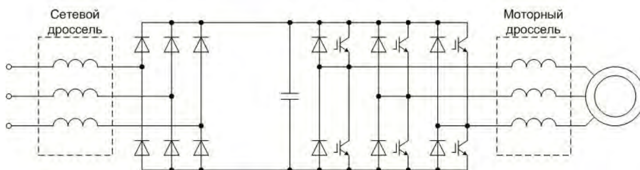
Схема подключения преобразователя частоты с сетевым и моторным дросселями.
