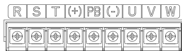
Схема силовых клемм AP2-300B и AP2-370B
